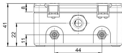
985 with cap nut conduit AF15
